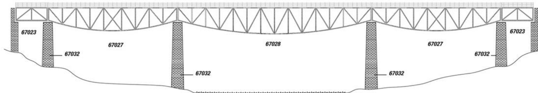
Kombinationsbeispiel: Fischbauchbrücken mit Vorflutern und Brückenfeilern (Gesamtlänge: 144 cm)
