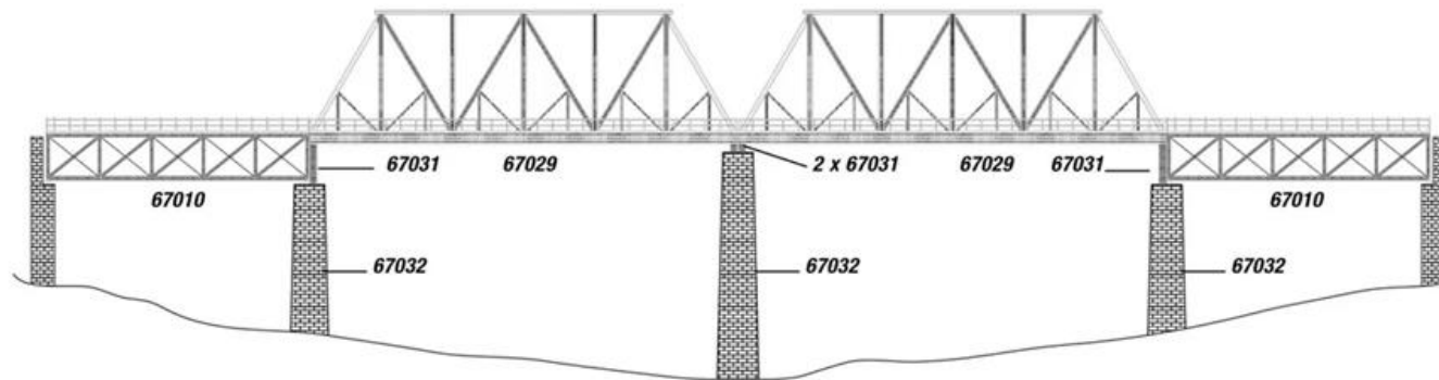
Kombinationsbeispiel: Kastenbrücken mit Stahlbrücken, Brückenfeilern und Adapterstücken (Gesamtlänge: 108 cm)
