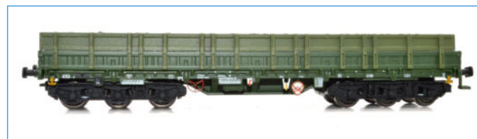
6-achsiger Schwerlastwagen Bauart Samms 4860 der DR (Epoche IV) erhöhte Bordwände, grün-grün-schwarz, beladen mit Kies NW 22233 H0 61,50 €
